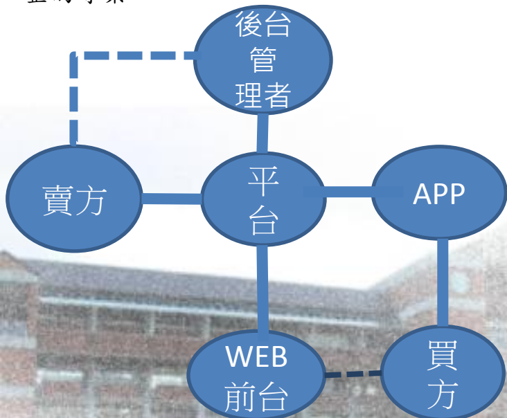
圖三、客戶端
